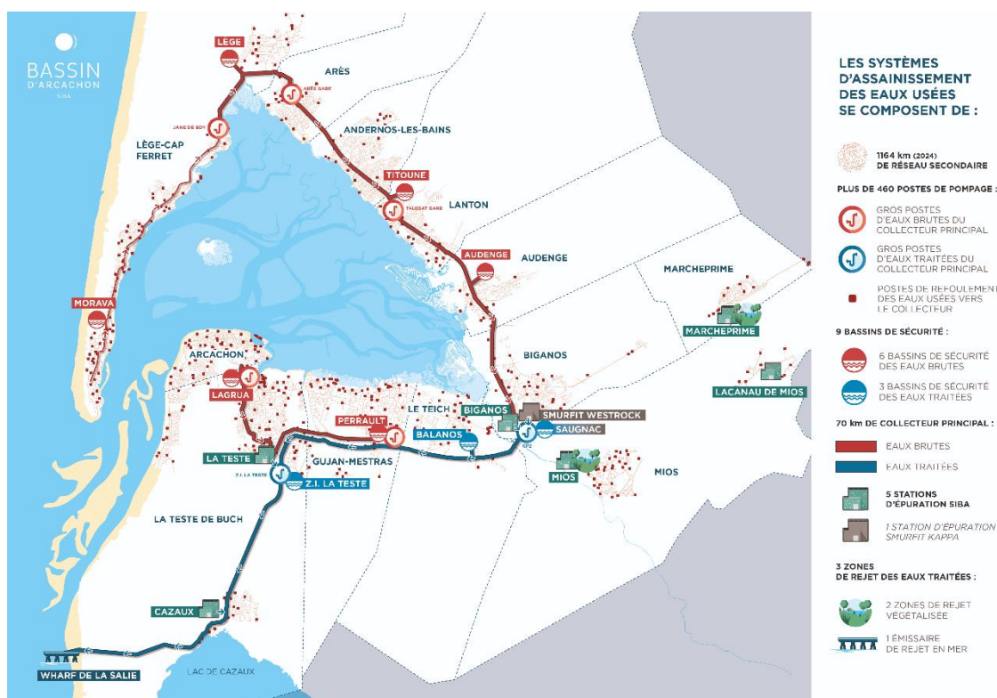
Figure 1 : Plan du réseau d'assainissement du Bassin d'Arcachon (SIBA)
